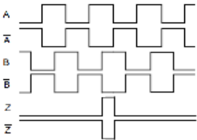
时序图
