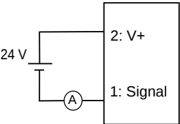
两线制电流
