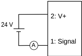
两线制电流
