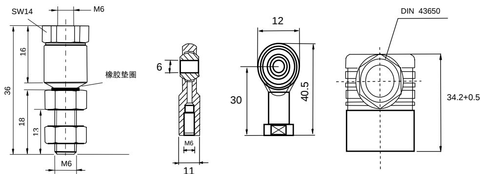
鱼眼接头
