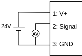
三线制电压/电流
